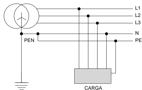
Figura 2 - Esquema TN-C-S
